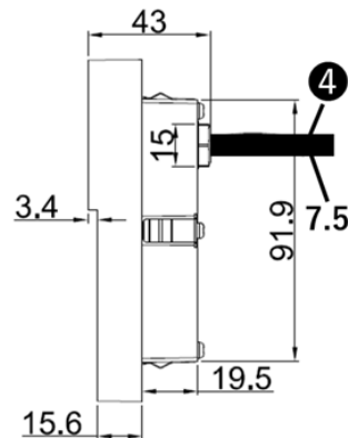
(灯具横面寸法)
