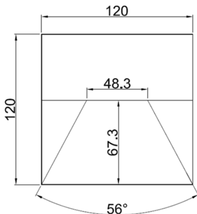
(灯具正面寸法)
