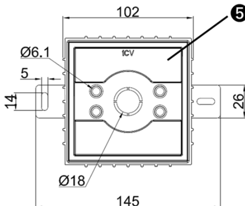
(ボックス正面寸法)
